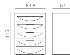
Elemento 5 cassetto P=57 H=115
