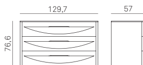
Elemento 3 cassetto P=57 H=76,6
