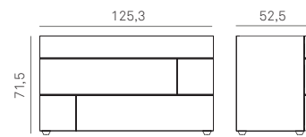
Elemento 3 cassetti P=52,5 H=71,5
