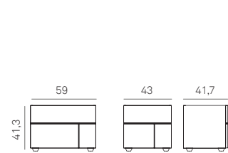
Elemento 2 cassetti P=41,7 H=41,3
