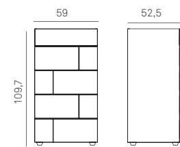
Elemento 5 cassetti P=52,5 H=109,7
