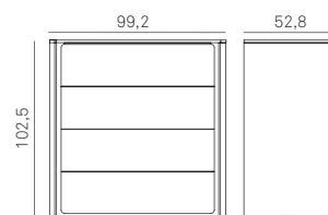
Elemento 4 cassette P=52,8 H=102,5
