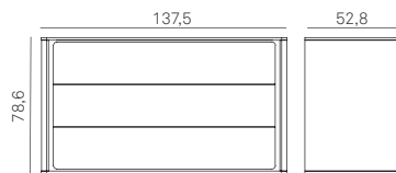
Elemento 3 cassette P=52,8 H=78,6
