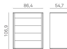
Elemento 5 cassetto P=54,7 H=106,9
