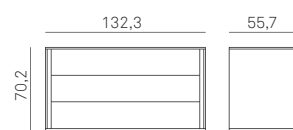
Elemento 3 cassetto P=54,7 H=70,2
