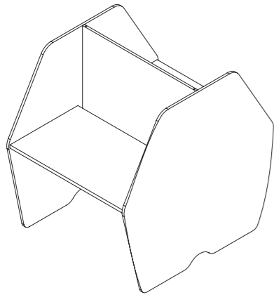
Fianchi per postazione singola/ Lateral side for single workstation P 67 H 131
